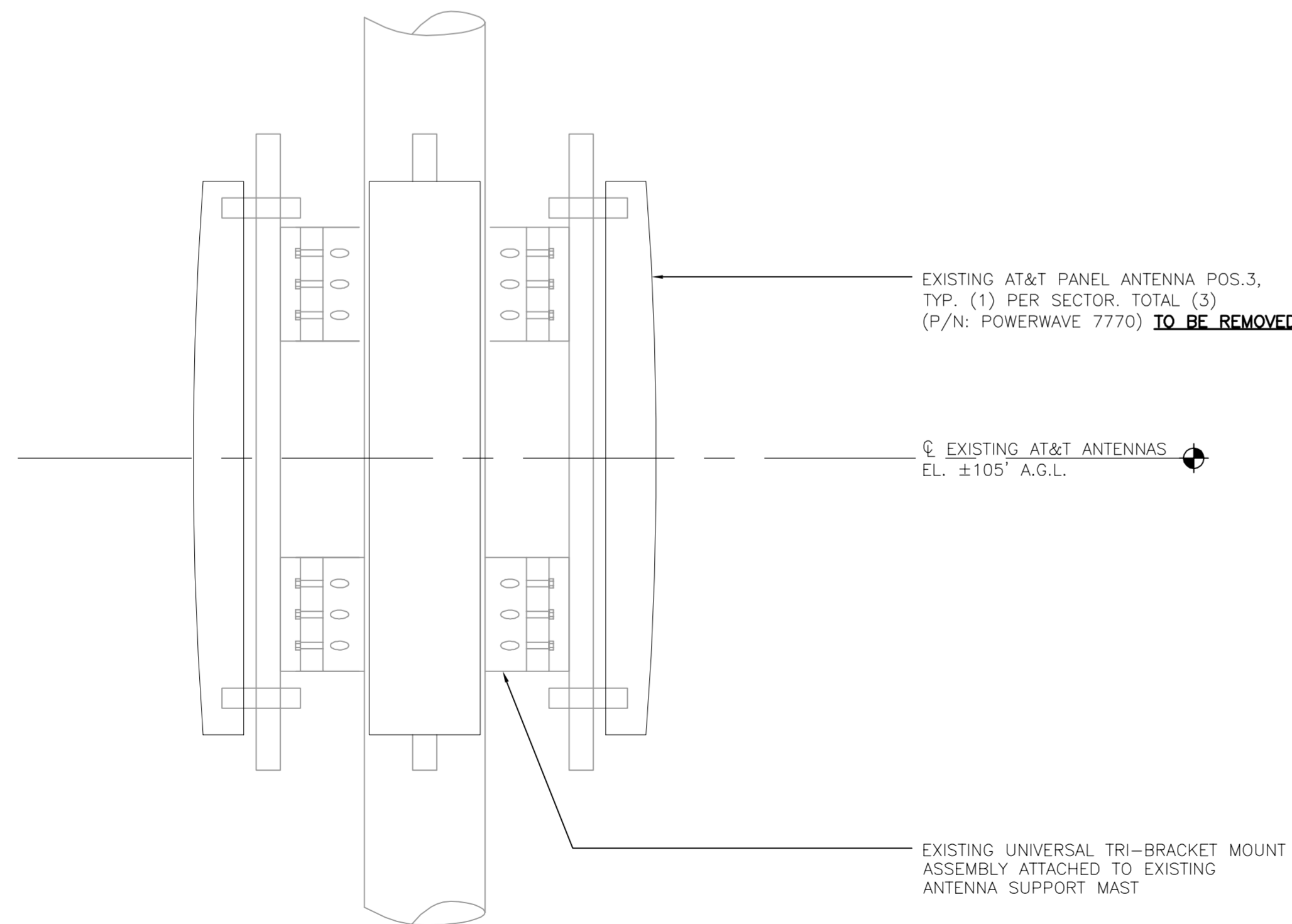
1A C-2 EXISTING ANTENNA ELEVATION SCALE: 1" = 1'-0"
