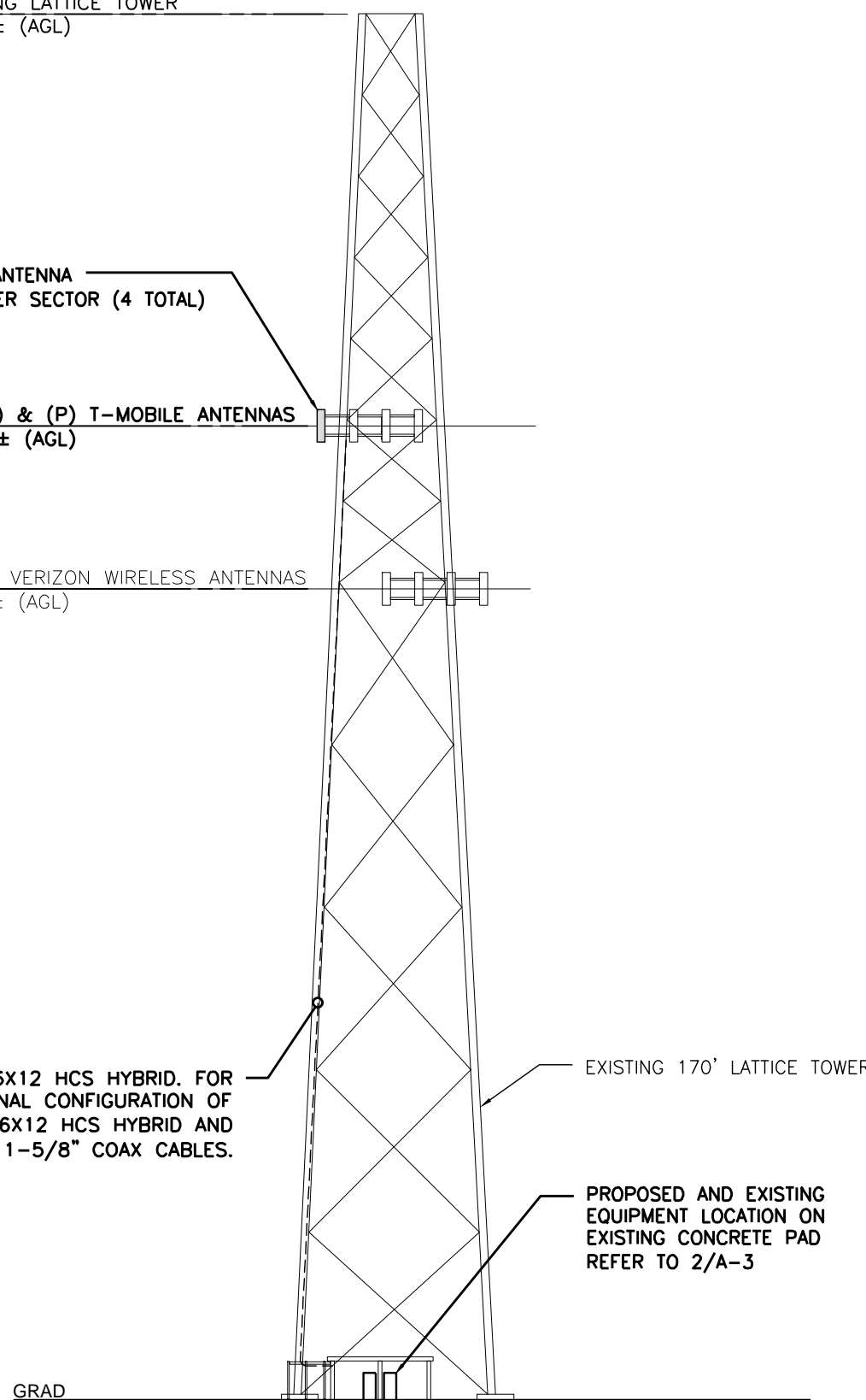
ELEVATION SCALE: 1" = 20'-0"
