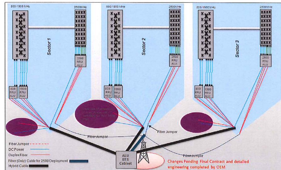
3 RAN WIRING A-5 SCALE: N.T.S.
