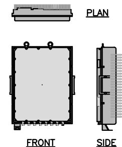
2500 MHz RRH DETAIL 3 SCALE: N.T.S. A-3
