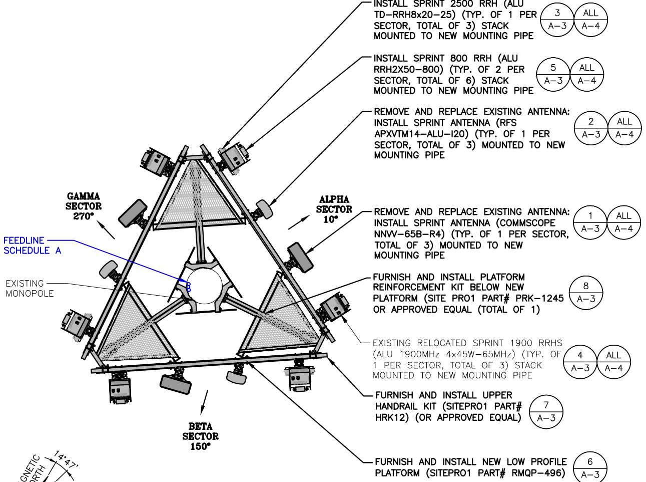
PROPOSED ANTENNA PLAN (2) A-2 22x34 SCALE: 3/8"=1'-0" 11x17 SCALE: 3/16"=1'-0"
