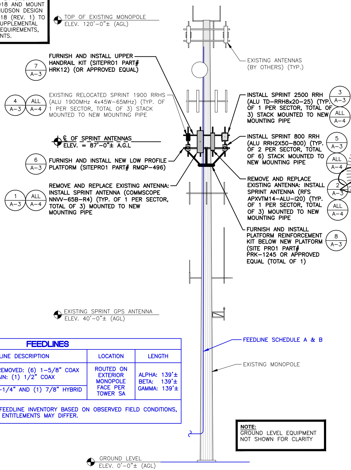
ELEVATION (3) A-2 22x34 SCALE: 1/8"=1'-0" 11x17 SCALE: 1/16"=1'-0"
