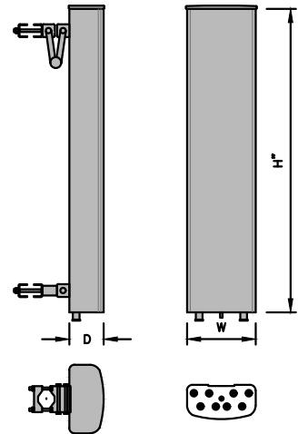
2500 MHZ ANTENNA DETAIL 2 SCALE: N.T.S. A-3
