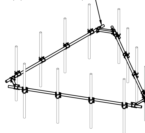
HANDRAIL KIT DETAIL 7 SCALE: N.T.S. A-3
