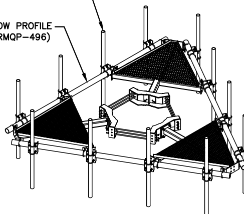
LOW PROFILE PLATFORM KIT DETAIL 6 SCALE: N.T.S. A-3
