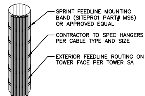
EXTERIOR FEEDLINE ROUTING 9 SCALE: N.T.S. A-3
