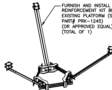
PLATFORM REINFORCEMENT KIT DETAIL 8 SCALE: N.T.S. A-3
