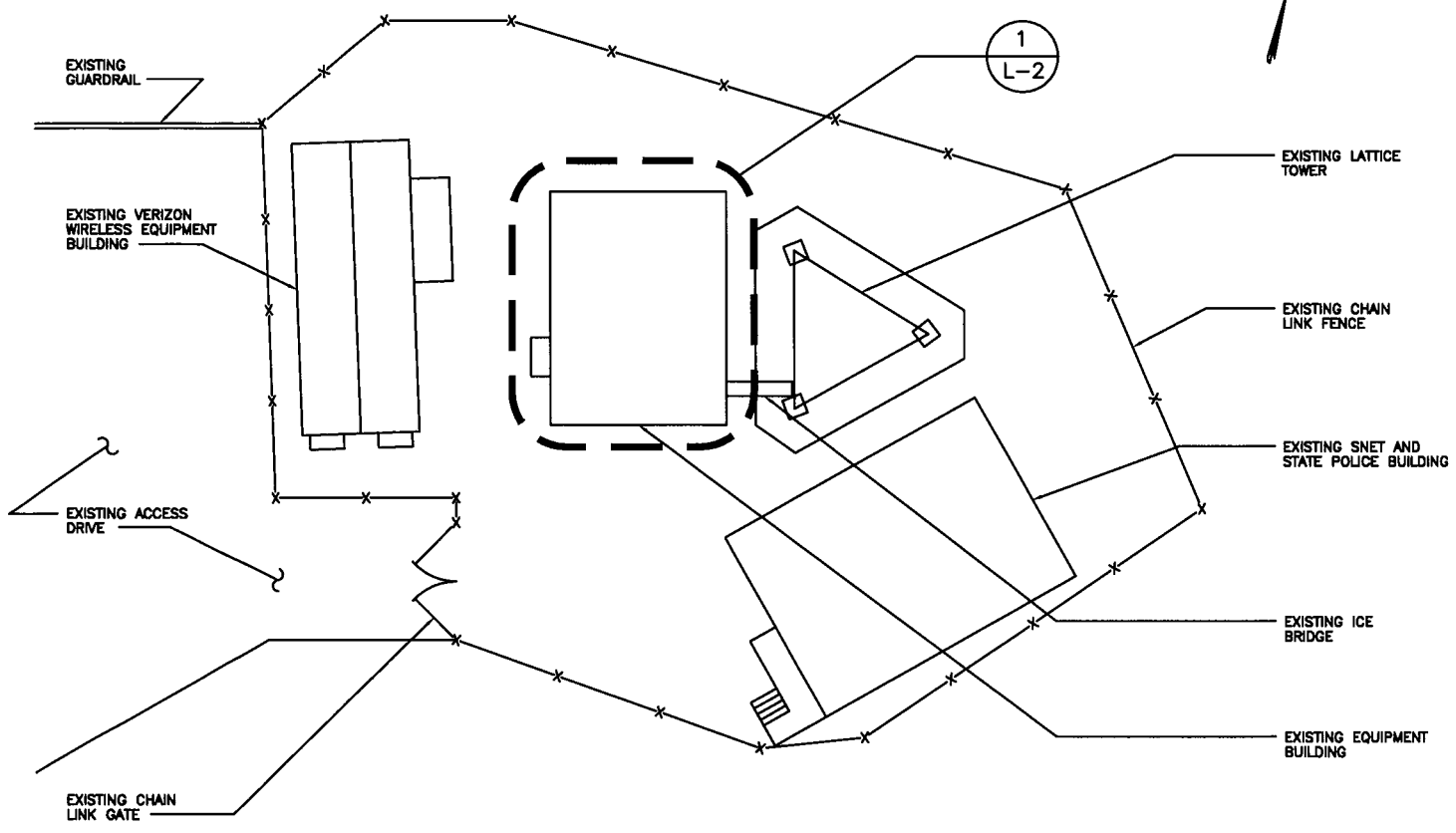
1 SITE PLAN L-1 SCALE: 1" = 20'-0"
