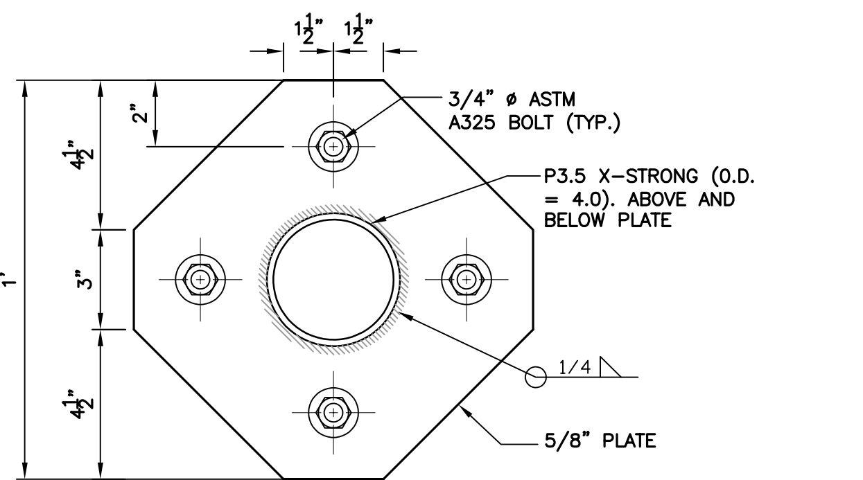
6 PLATE 'P2' DETAIL S-1 SCALE: 3" = 1'-0"
