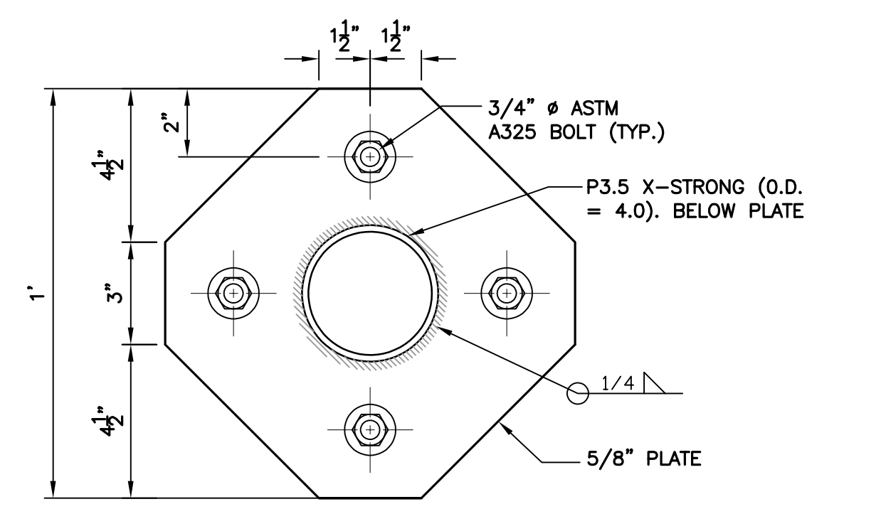
7 PLATE 'P3' DETAIL S-1 SCALE: 3" = 1'-0"
