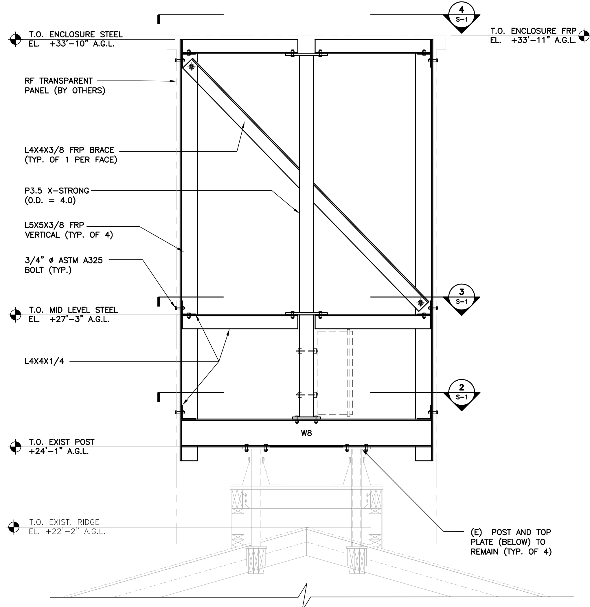
1 ENCLOSURE ELEVATION S-1 SCALE: 3/4" = 1'-0"
