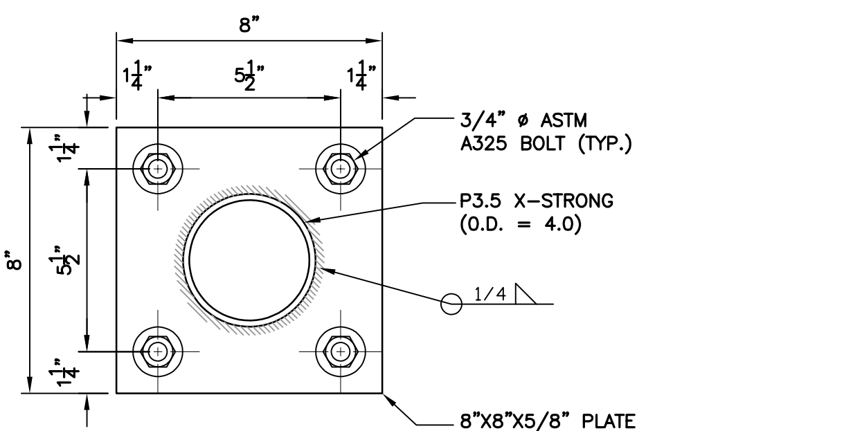
5 PLATE 'P1' DETAIL S-1 SCALE: 3" = 1'-0"
