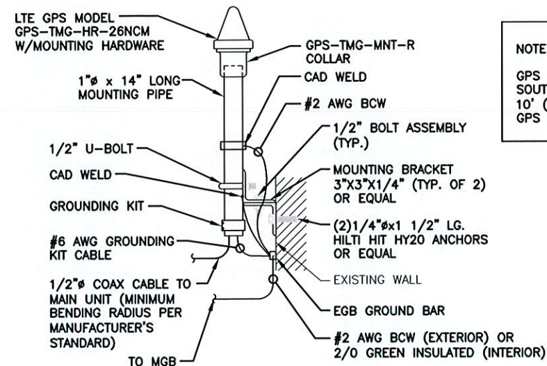
GPS MOUNTED TO WALL SCALE: N.T.S.
